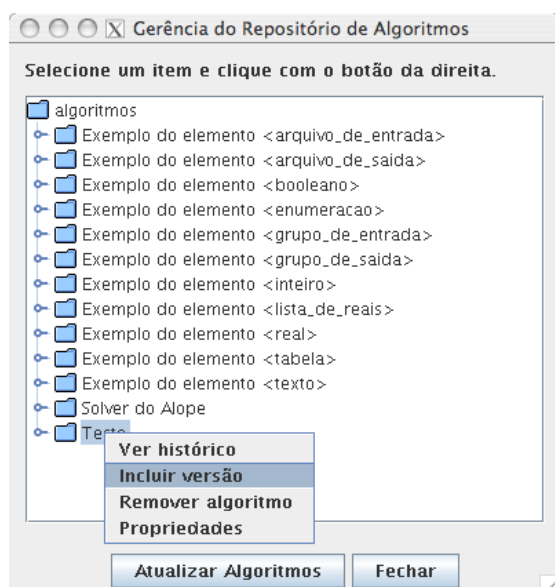
Figura 6: Incluir Versão do Algoritmo
